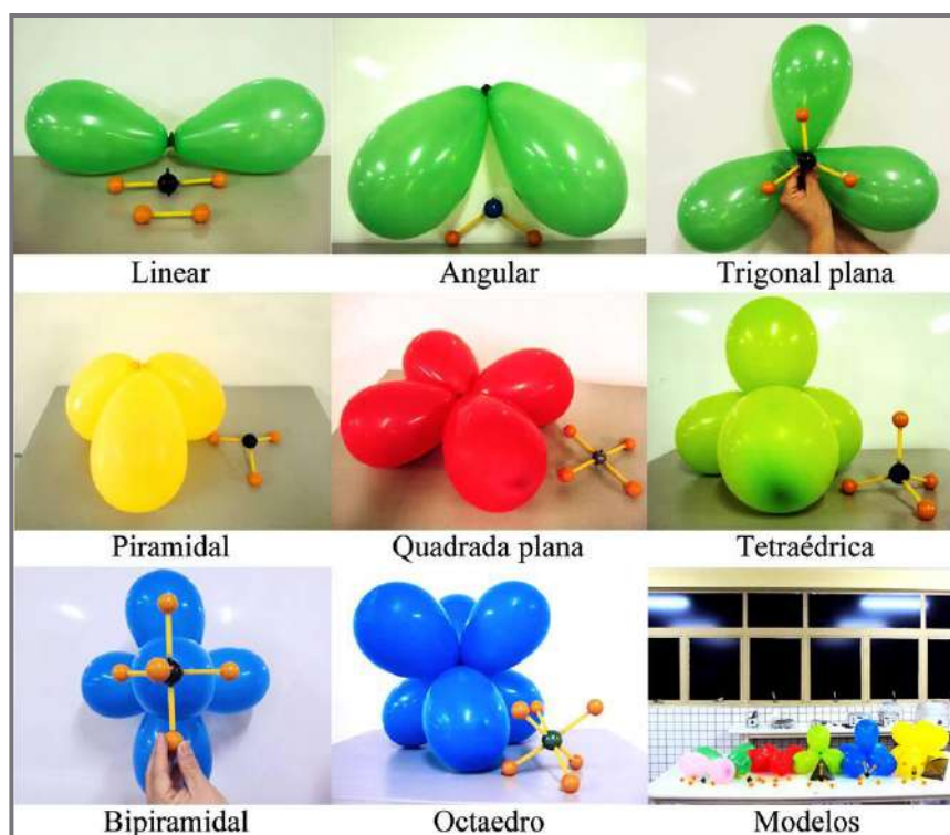
Figura 6 - Geometria Molecular com balões e bolas/bastões
