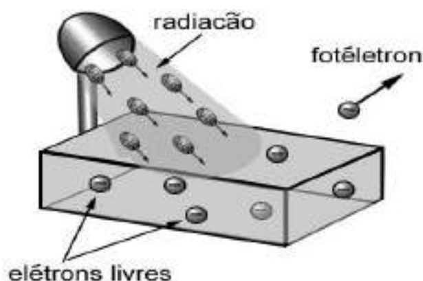
Figura 3; Efeito fotoelétrico.
