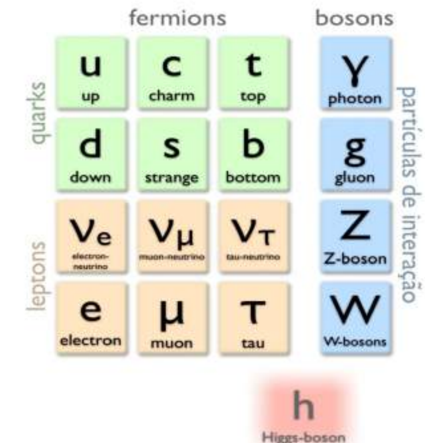
Figura 9; Classificação das partículas.
