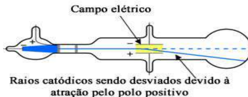
Figura; 2 Experimento de Thomson com tubo de raios catódicos
