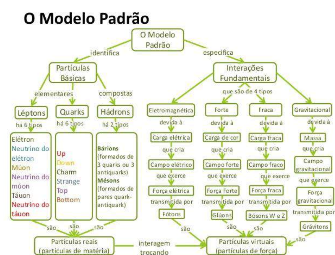
Figura 10; Modelo Padrão
