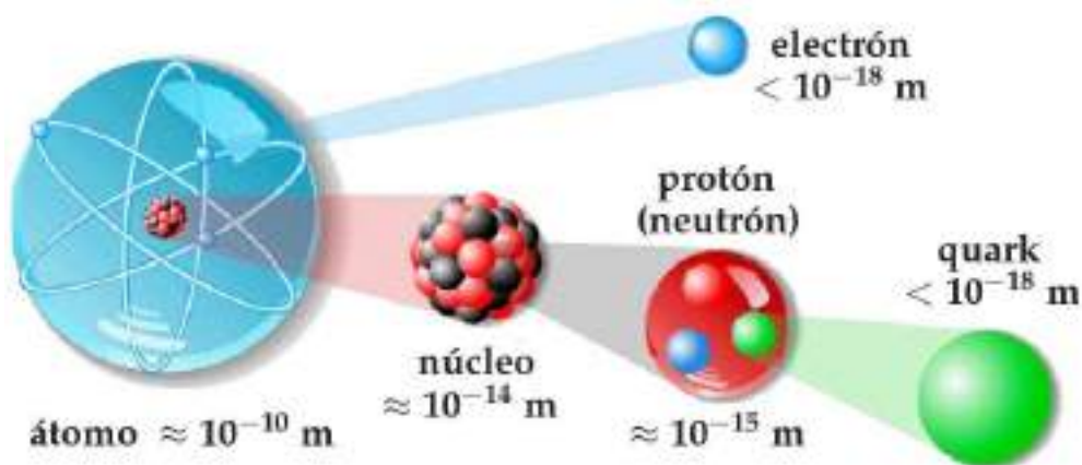
Figura 8; Do átomo ao quark
