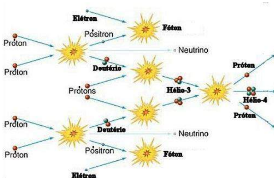
Figura 6; Neutrino
