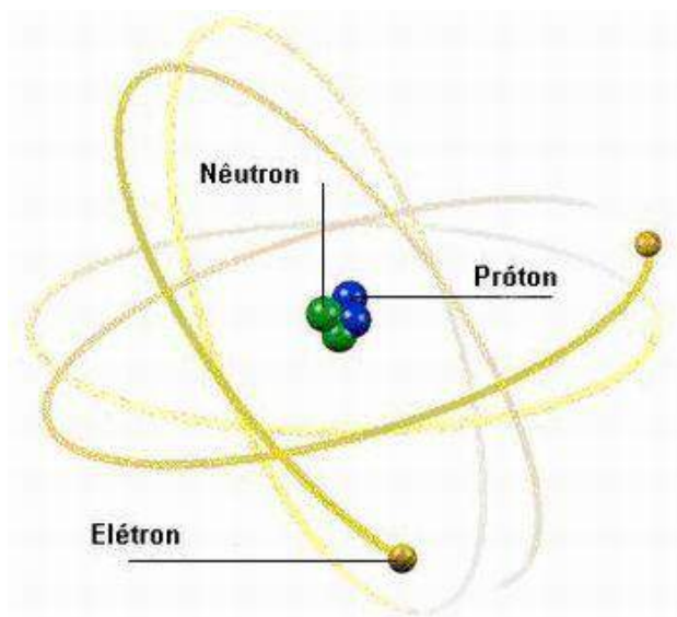
Figura 1; Modelo Atômico
