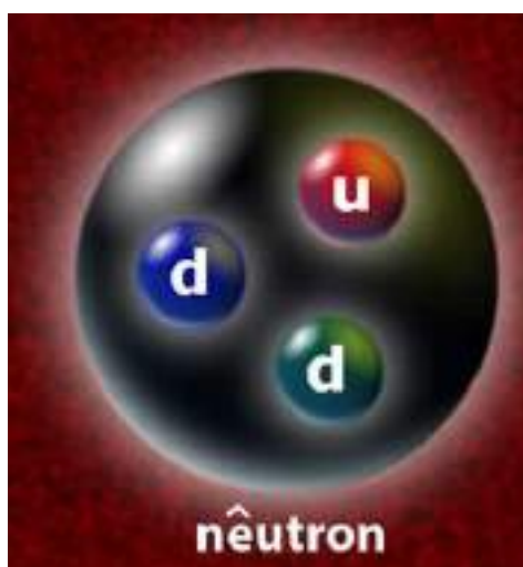
Figura 5; Nêutron /partícula subatômica formada por três partículas (udd) denominada quarks
