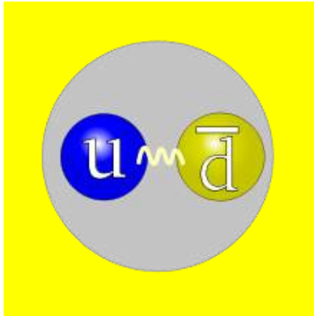
Figura 8 Píon
