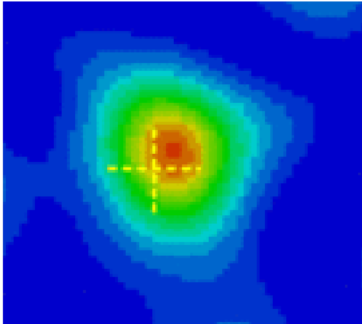
Figura 7; Múon
