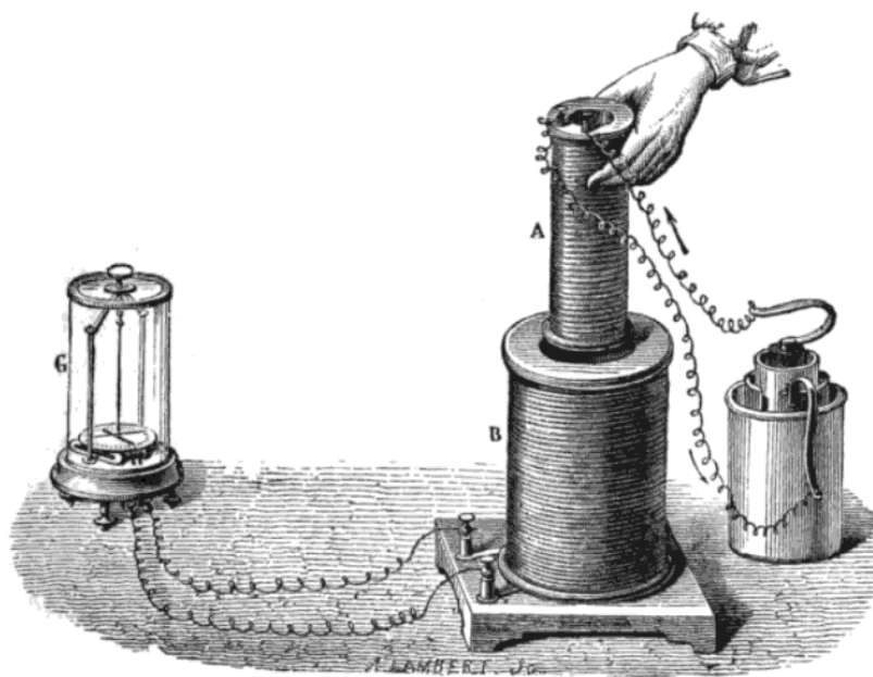
Figura 13 - Representação do experimento de Faraday. Uma bateria (à direita) fornece uma corrente que atravessa um pequeno rolo de arame com núcleo de ferro (A), criando um eletroímã. Quando a bobina pequena é movida para dentro ou para fora da grande bobina (B), uma corrente é detectada pelo galvanômetro (L). Fonte: https://en.wikipedia.org/wiki/File:Induction_experiment.png .
