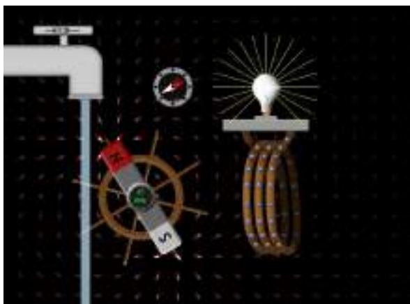
Figura 49 - Simulação do gerador. Fonte: https://phet.colorado.edu/pt_BR/simulation/generator
