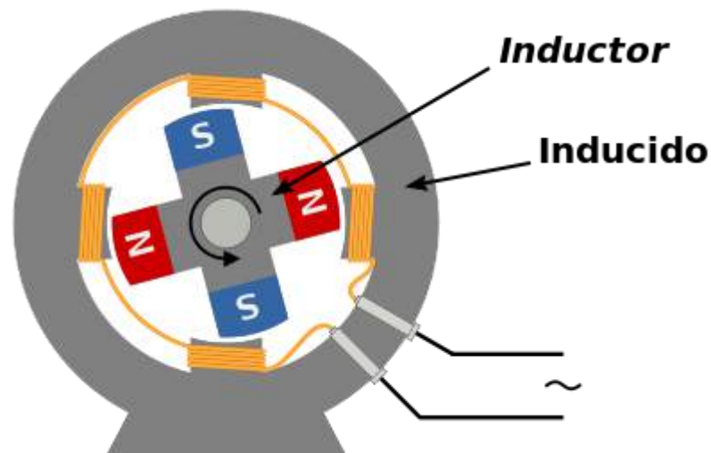
Figura 15 - Esquema de um alternador - Fonte: https://commons.wikimedia.org/wiki/File:Alternador.svg
