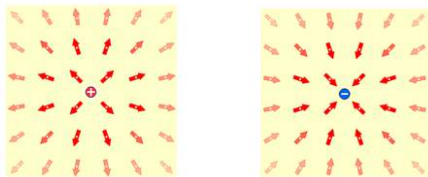
Figura 9 - Representação de Campos Elétricos
