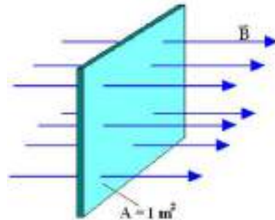
Figura 18 - Linhas de campo magnético atravessando uma superfície plana - Fonte: http://www.mundoeducacao.com/fisica/fluxo-magnetico.htm
