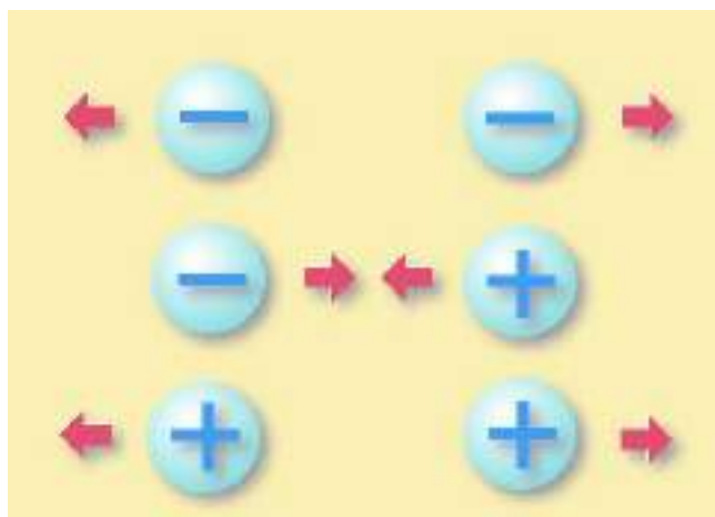
Figura 10 - Atração e repulsão em função do tipo de carga dos portadores (fonte: wikimedia commons)
