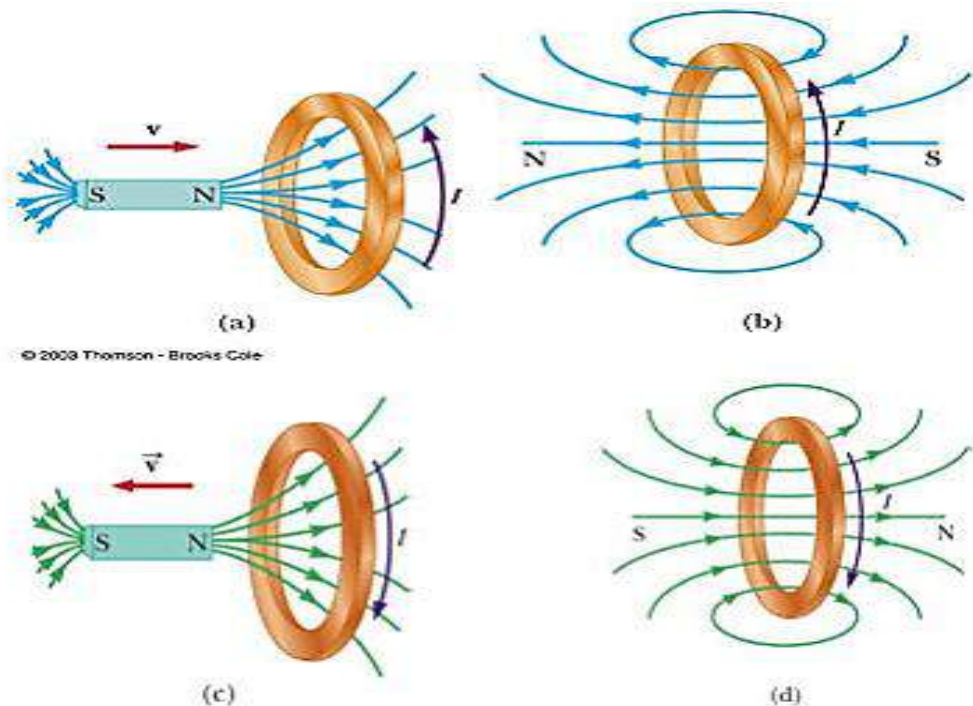
Figura 21 - Ilustração da Lei de Lenz - Fonte: http://objetoseducacionais2.mec.gov.br/bitstream/handle/mec/12613/05_teorias_frame.htm
