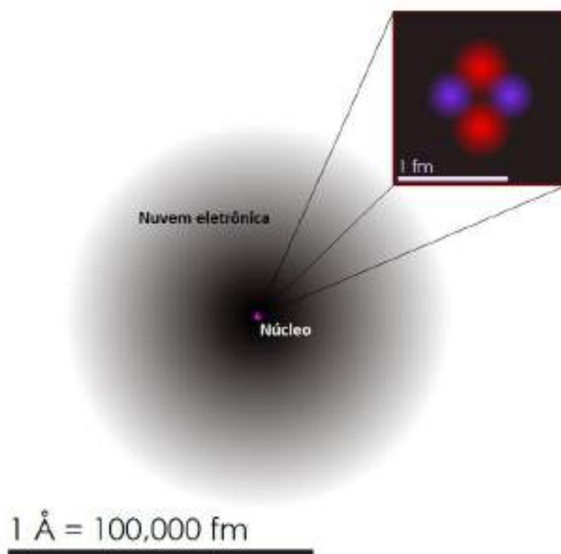
Figura 7 - Modelo mecânico-quântico - Fonte: https://commons.wikimedia.org/wiki/File:Helium_atom_QM.svg
