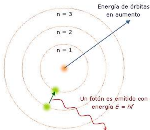
Figura 5 - Modelo de Bohr - Fonte: https://commons.wikimedia.org/wiki/File:Modelo_de_Bohr.png?uselang=pt-br
