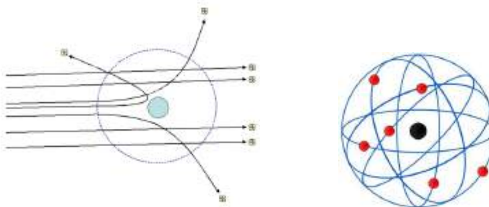
Figura 4 - A interpretação de Rutherford para os desvios observados (à esquerda), lhe permitiu conceber o modelo com núcleo positivo cercado de elétrons (à direita). Fonte: https://commons.wikimedia.org
