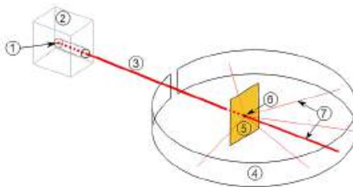
Figura 3 - Experimento da folha de ouro. 1: fonte radioativa (polônio), 2: blindagem de chumbo, 3: feixe de partículas alfa, 4: tela fluorescente ou filme fotográfico, 5: folha de ouro, 6: ponto em que o feixe de partículas atinge a folha, 7: algumas partículas são desviadas em relação ao feixe original. - Fonte: https://commons.wikimedia.org/wiki/File:Rutherford_Scattering.svg
