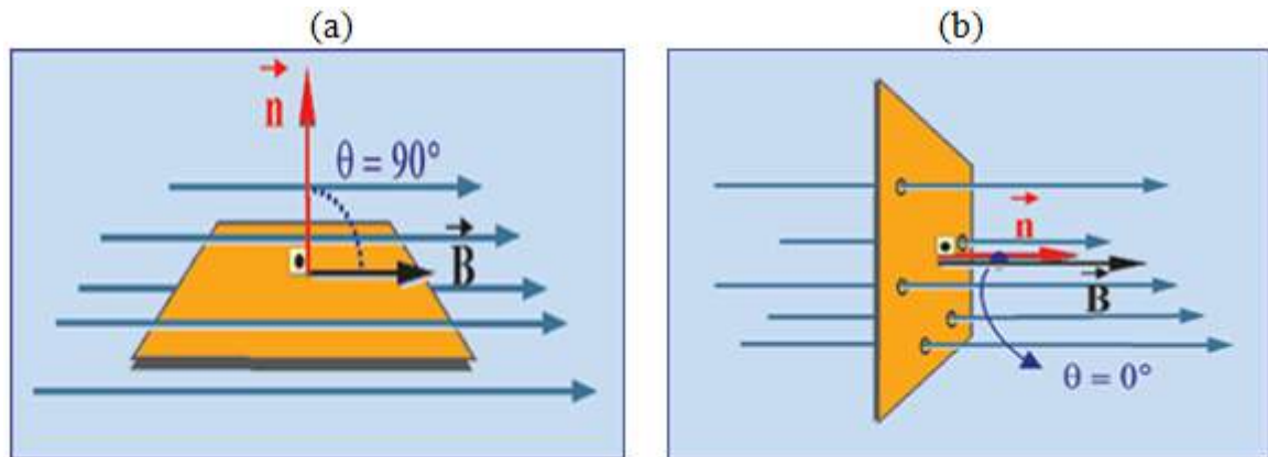
Figura 20 (a) e (b) - Conceito de fluxo magnético. Fonte: http://interna.coceducacao.com.br/ebook/pages/9734.htm
