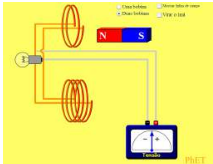
Figura 50 - Simulação da lei de Faraday – Fonte: https://phet.colorado.edu/sims/faradays-law/faradays-law_pt_BR.html
