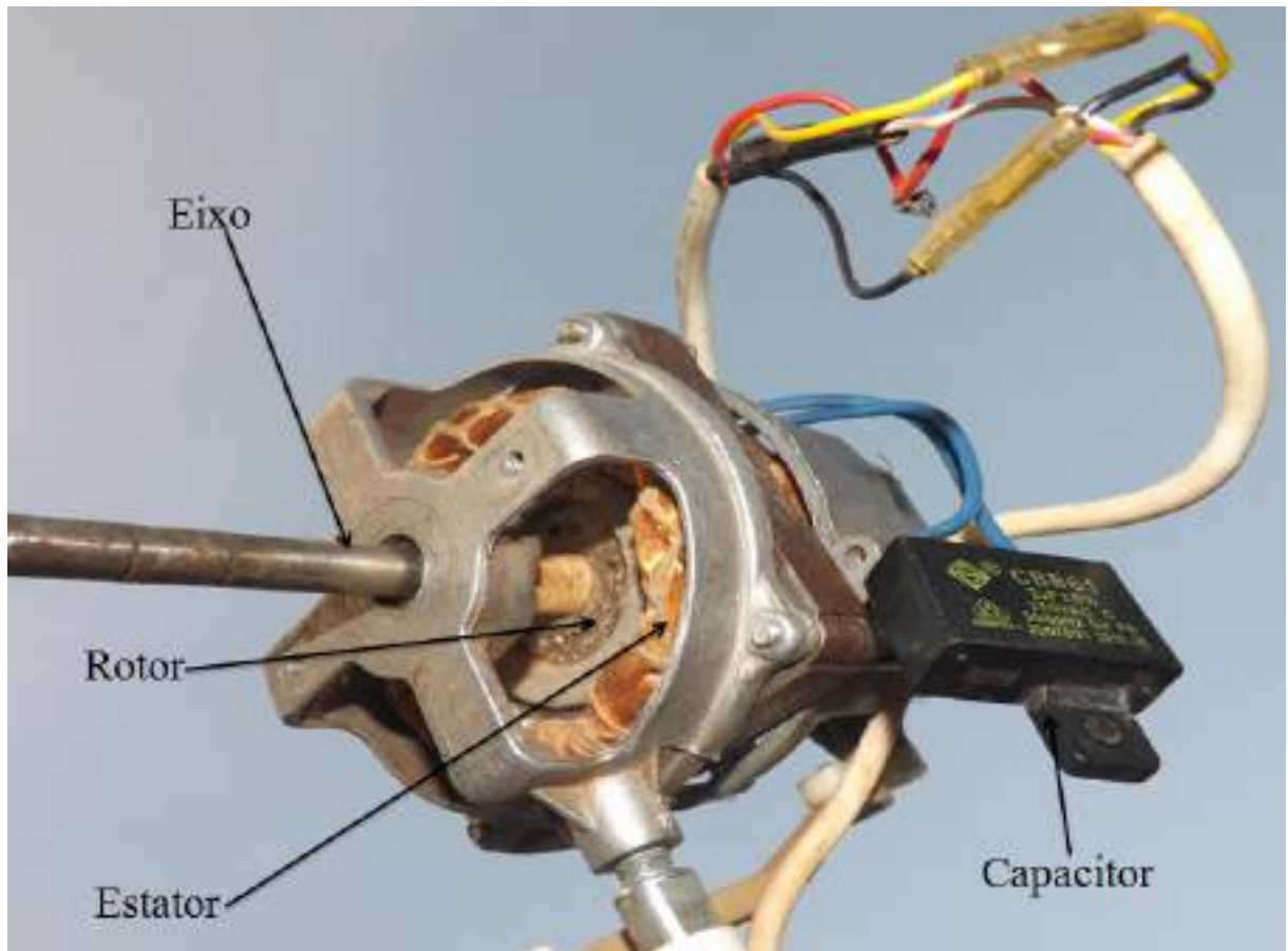
Figura 31 - Partes do motor de ventilador
