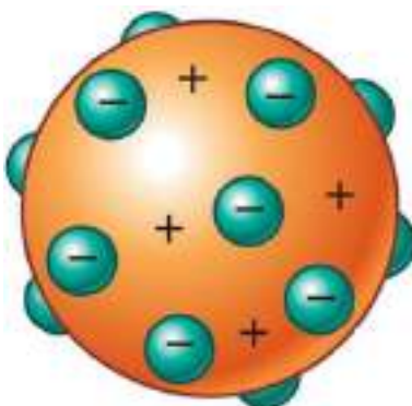
Figura 2 - Modelo de Thomson - Fonte: http://www.brasilecola.com/quimica/o-experimento-thomson-com-descargas-eletricas.htm
