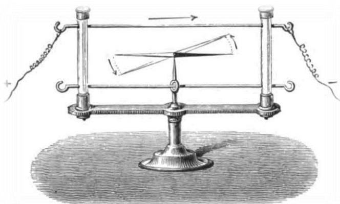
Figura 12 - Representação da experiência de Oersted - Fonte: https://en.wikipedia.org/wiki/File:Oersted_experiment.png .
