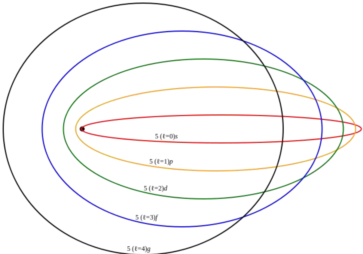
Figura 6 - Representação do modelo atômico de Sommerfeld - Fonte: https://commons.wikimedia.org/wiki/File:Sommerfeld_ellipses.svg
