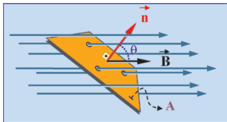
Figura 19 - Conceito de fluxo magnético - Fonte: http://interna.coceducacao.com.br/ebook/pages/9733.htm
