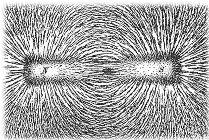
Figura 17 - Campo magnético de um ímã em forma de barra que foi coberto por uma folha de papel. Ao polvilhar limalha de ferro sobre o papel, os fragmentos se alinham sob a influência do referido campo. Fonte: https://commons.wikimedia.org/wiki/File:Magnet0873.png
