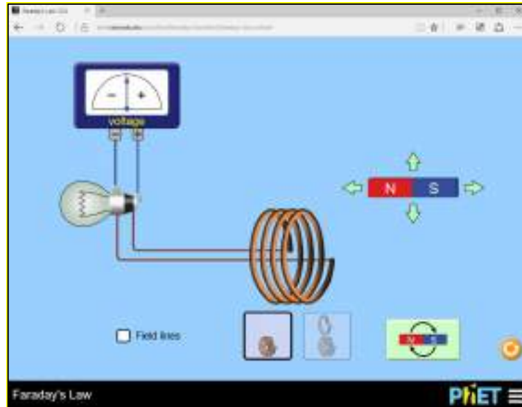
Figura 14 - Simulação interativa que ilustra o fenômeno da indução a partir do movimento relativo entre ímã e espira. Fonte: PHET / University of Colorado.
