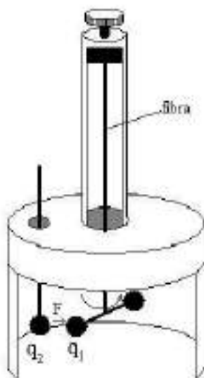
Figura 8 - Balança de Torção - Fonte: https://pt.wikibooks.org/wiki/Eletromagnetismo/Cargas_el%C3%A9tricas
