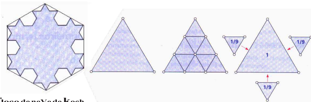
floco de neve de Koch
